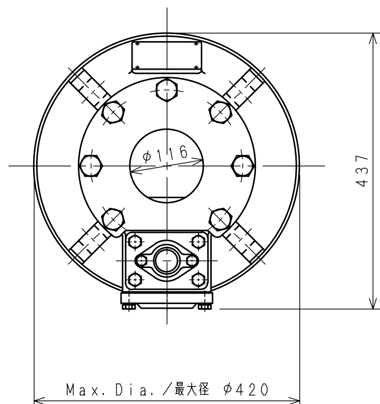
100A Companion Flange 100A 溶接用相フランジ
