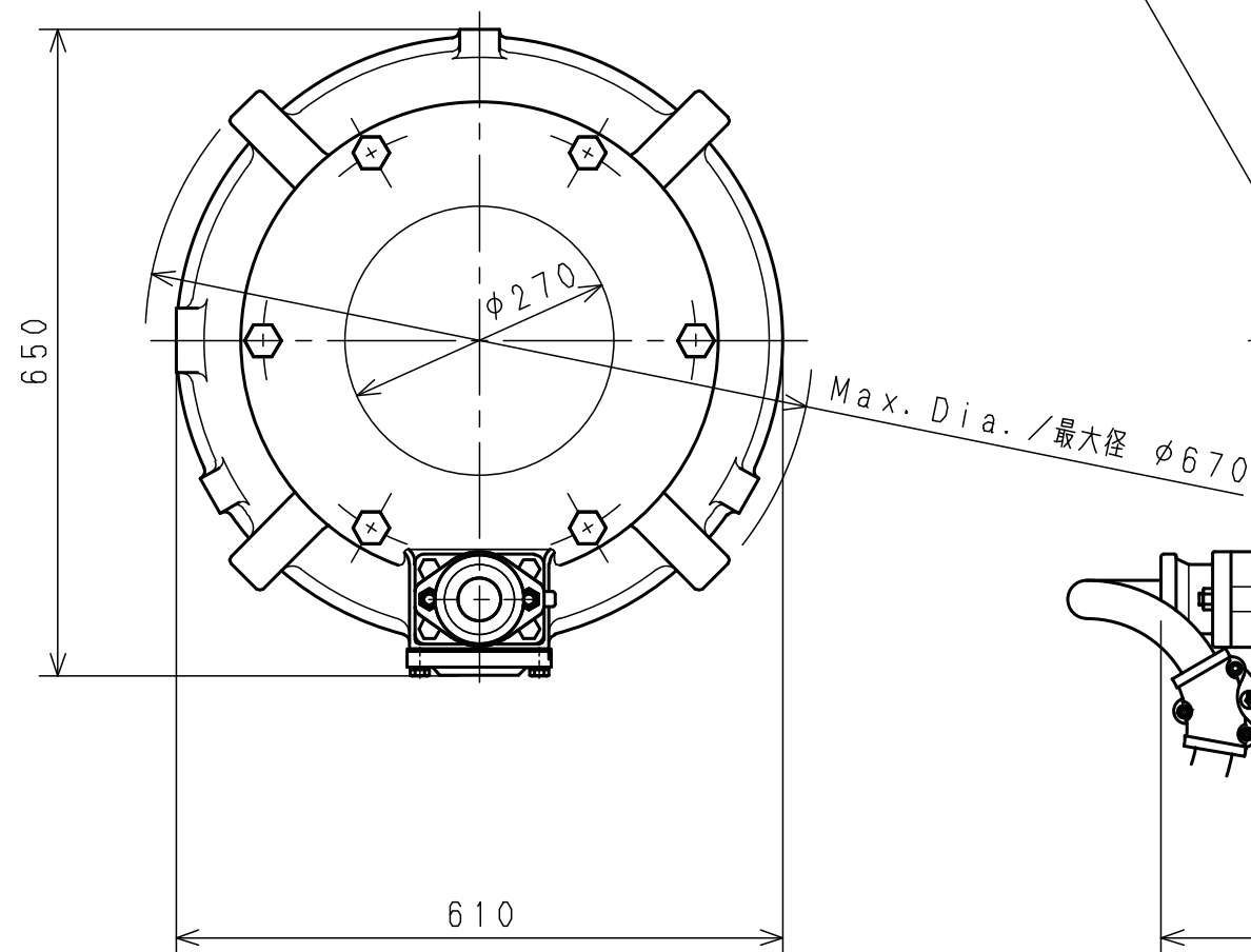
250A Companion Flange 250A 溶接用相フランジ
