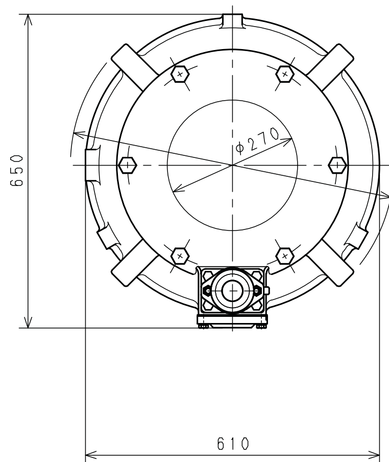
Max. Dia. / 最大径 \phi 670
