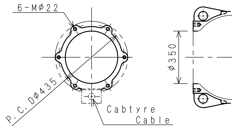
Flange Dimension フランジ寸法
