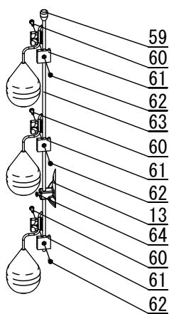
フロートスイッチ詳細図
