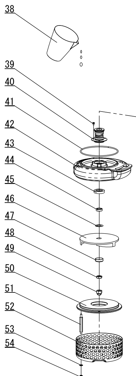
フロートスイッチ詳細図
