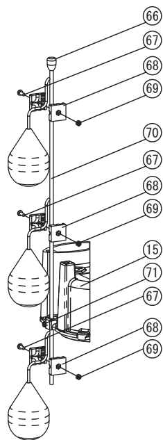
フロートスイッチ詳細図
